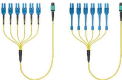
Singlemode OS2
